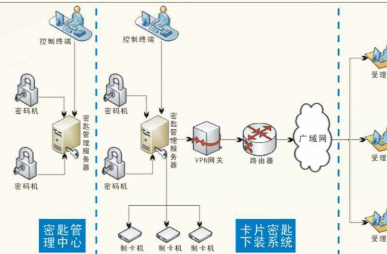
卡德密钥管理系统拓扑图
