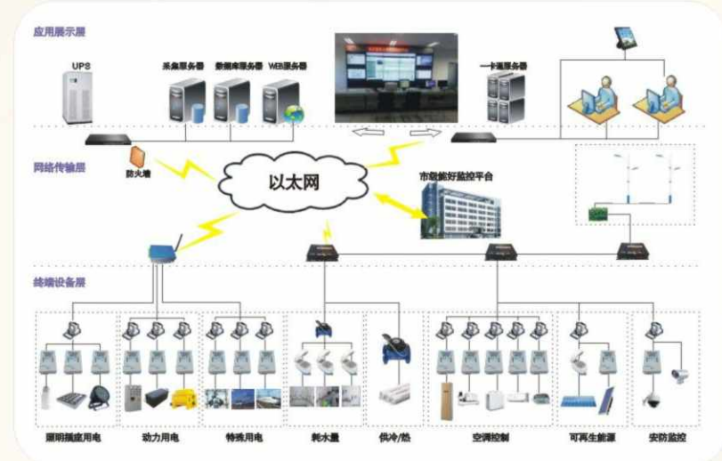
节能监管综合服务平台网络架构
